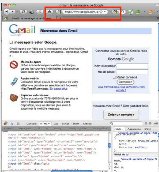
Lors d'une attaque avec l'outil SSLStrip tous les liens sont alors convertis en HTTP
