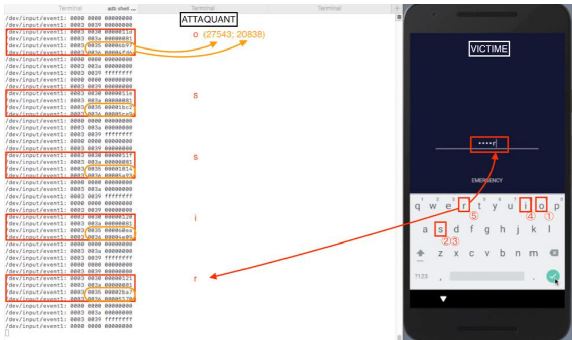
Évènements de déverrouillage du téléphone retournés par la commande getevent
