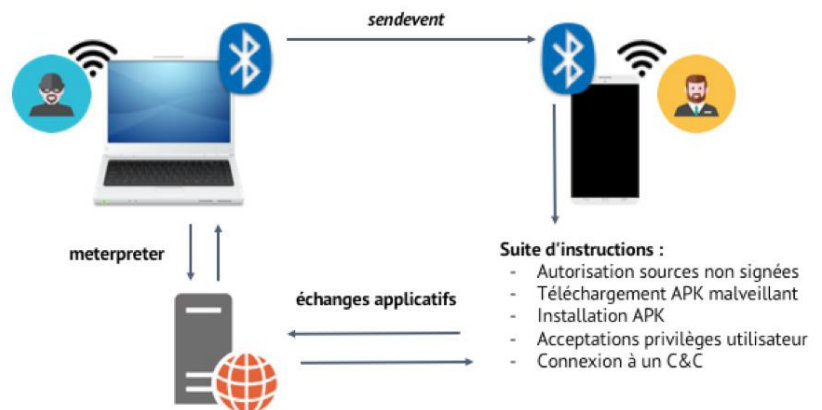
Principes du scénario de post-exploitation 'Installation d'une application malveillante'
